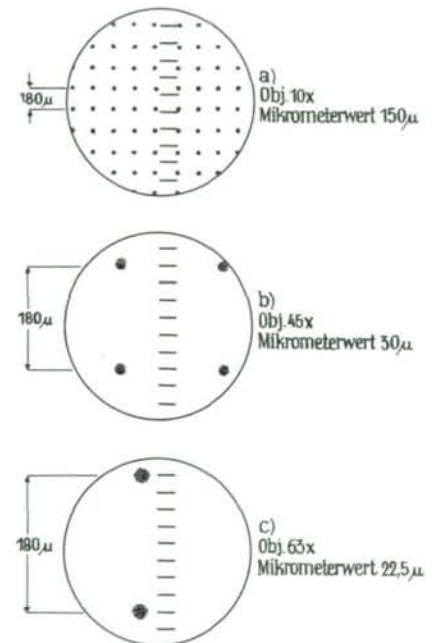
Abb. 2: Bestimmen der Mikrometerwerte verschiedener Objektive (siehe Text).
