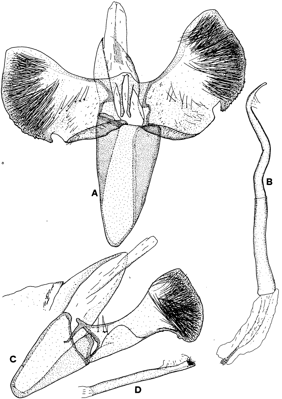
PLATE V. A - B: Aspilapteryx magna n.sp. A: Male genitalia; B: Aedeagus. – C - D: A. seriata MEYR. C: Male genitalia; D: Aedeagus.
